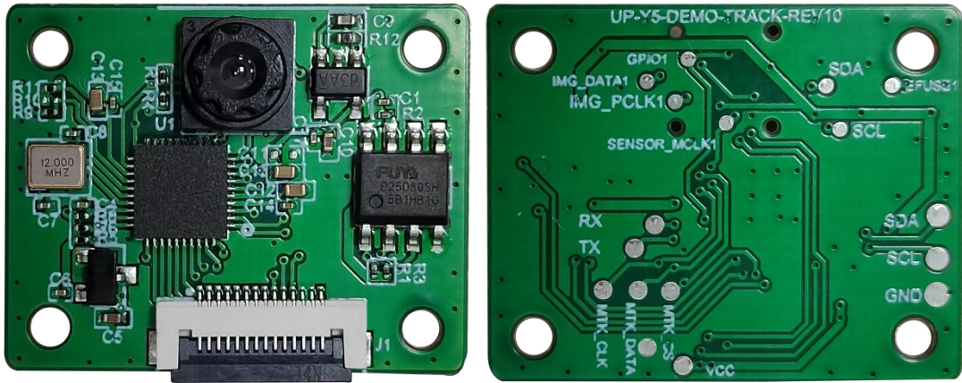
图 1 模块结构图
